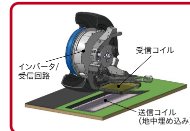
● 走行中ワイヤレス給電 第3世代ワイヤレスインホイールモータ
