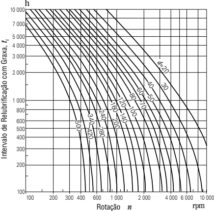
(2) Rolamentos de Rolos Cônicos, Rolamentos Autocentradores de Rolos
