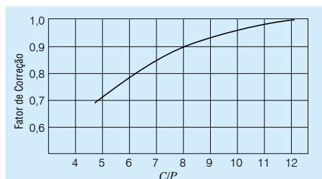
Fig. 6.1 Correção do Limite de Rotação devido à Intensidade da Carga no Rolamento
