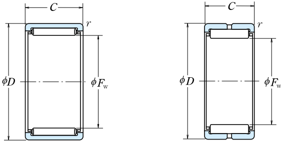
Sem anel Interno
