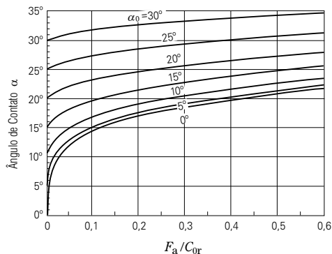
Fig. 15.1 F_a/C_{0r} e o Ângulo de Contato dos Rolamentos Fixos de Esferas e Rolamentos de Contato Angular
