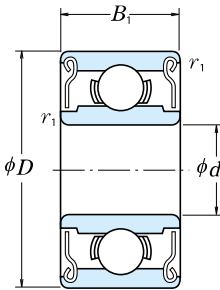
Blindado ZZ - ZZ1
