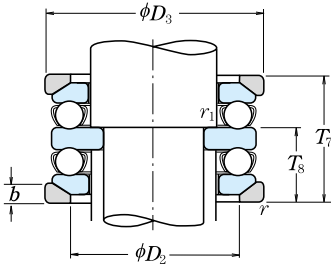
Com Contraplaca Esférica
