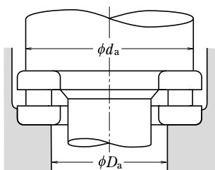
Fig. 11.4 Diâmetro da Superfície de Suporte do Rolamento Axial de Roos
