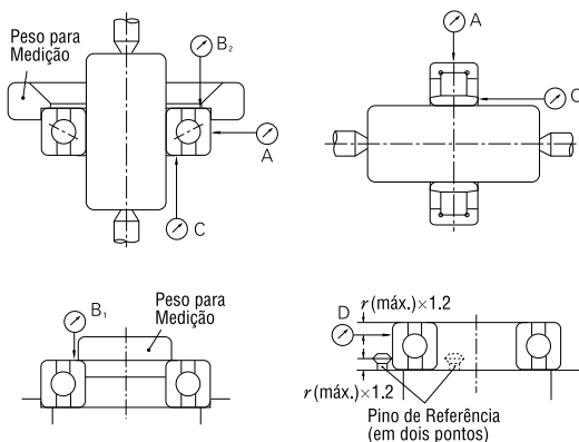
Fig. 8.1 Métodos de Medição da Precisão de Giro (simplificado)
