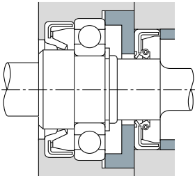
Fig. 11.8 Exemplo de Retentores (1)
