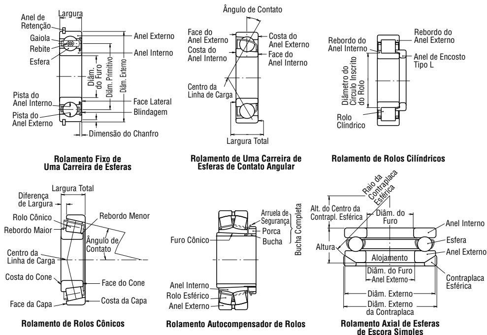
Fig. 1.1 Designação das Partes dos Rolamentos
