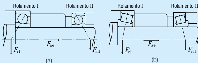
Fig. 5.12 Cargas Atuantes nos Rolamentos Contrapostos
