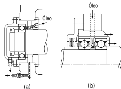
Fig. 12.8 Lubrificação por Jato
