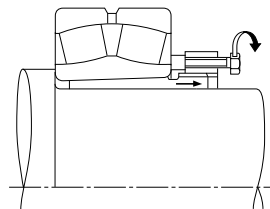
Fig. 14.17 Remoção da Bucha de Desmontagem (2)
