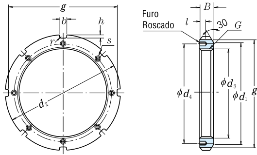
Porca para Uso com Grampo
