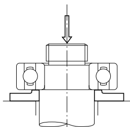
Fig. 14.12 Remoção pelo Anel Interno com Prensa
