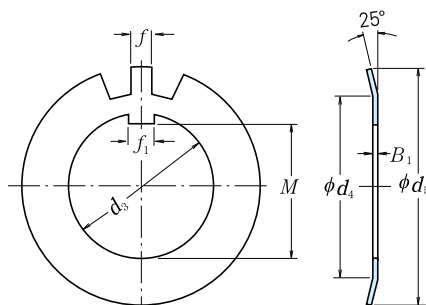
Aba Interna Reta
