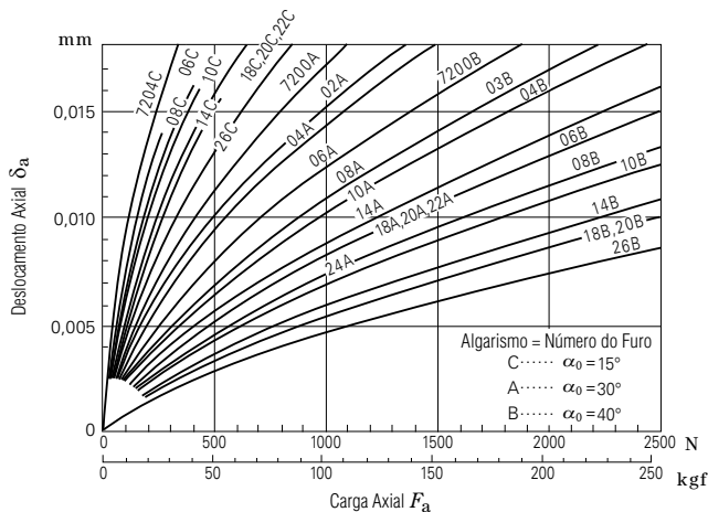
Fig. 15.3 Carga Axial e o Deslocamento Axial dos Rolamentos de Esferas de Contato Angular
