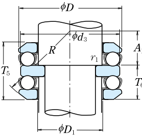
Com Assento Esférico
