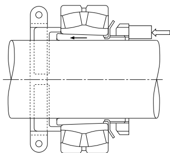
Fig. 14.18 Remoção da Bucha de Fixação
