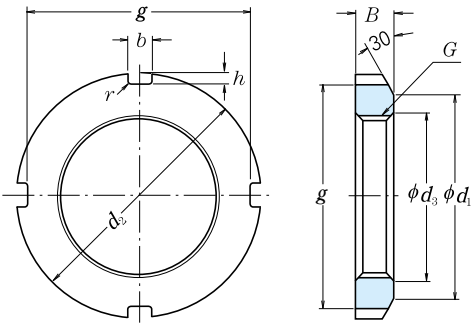
Porca para Uso com Arruela
