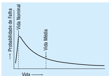
Fig. 5.2 Dispersão da Vida do Rolamento
