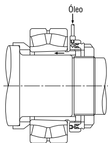
Fig. 14.6 Instalação com Porca Hidráulica
