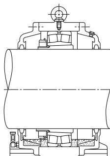
Fig. 12.4 Lubrificação por Banho de Óleo
