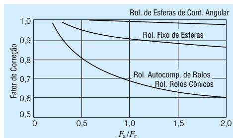
Fig. 6.2 Correção do Limite de Rotação devido à Carga Combinada
