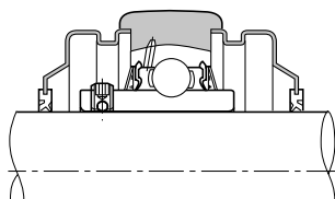
Fig. 2.2 Tampa de Aço Estampado
