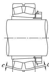
Fig. 14.8 Medição de Folga no Rolamento Autocompensador
