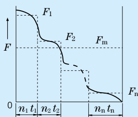
Fig. 5.7 Carga de Variação Escalonada
