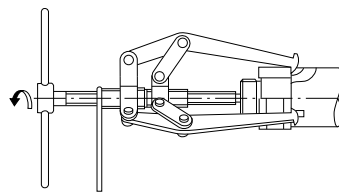
Fig. 14.14 Remoção do Anel Interno com Extrator (2)
