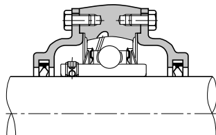
Fig.2.3 Tampa de Ferro Fundido
