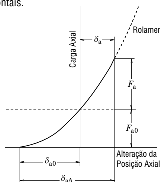
Fig. 10.5 Deslocamento Axial no Pré-carregamento de Pressão Constante
