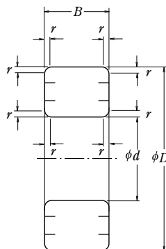
Fig. 7.1 Dimensões Principais dos Rolamentos Radiais de Esferas e de Rolos
