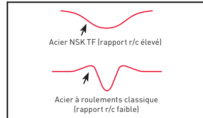
Réduction des contraintes au bord des indentations lors de la contamination
