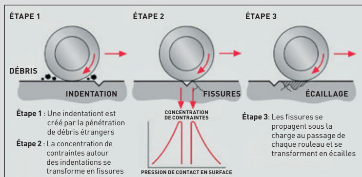
Écaillage en surface dans les environnements contaminés
