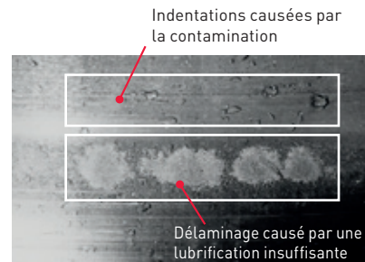
Dureté et résistance à l'usure supérieures des pistes de roulement
